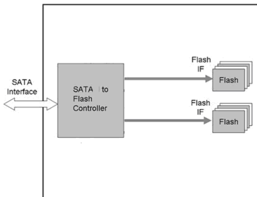
Figure 1-1 Apacer mSATA Mini M4-M block diagram
