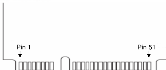
Figure 1-2 Apacer mSATA Mini M4-M pin assignment
