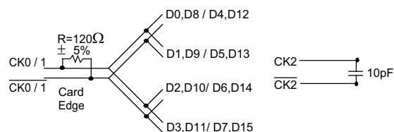
*Clock Net Wiring
